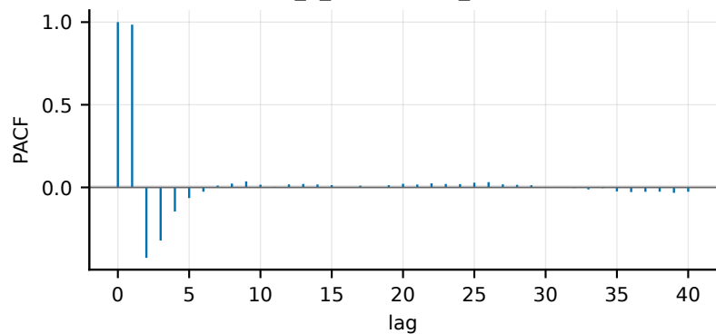
DO_1_1 (autocorr_aware)
