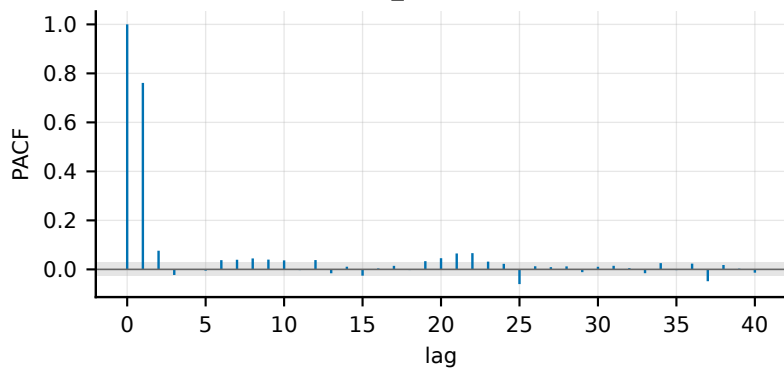
inf_COD (iid)
