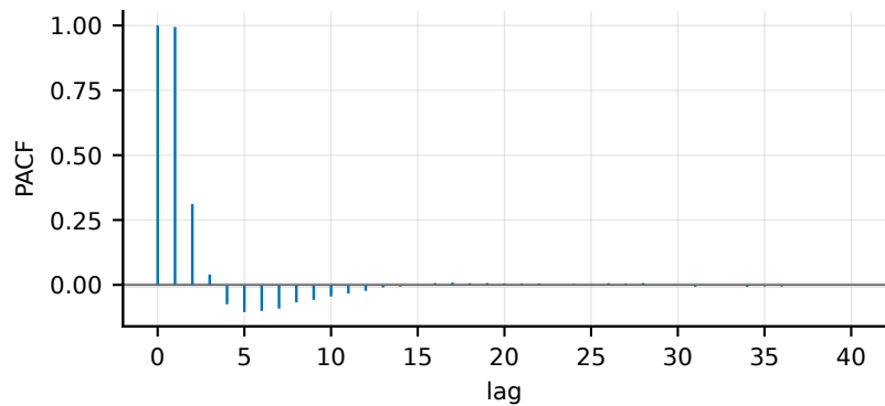
DO_1_1 (autocorr_aware)
