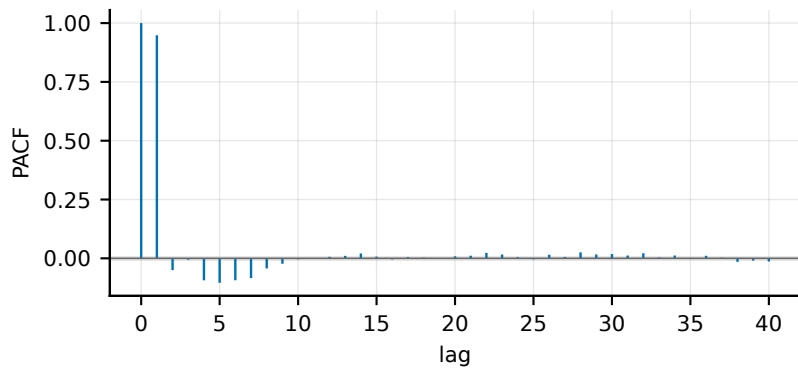
inf_COD (iid)
